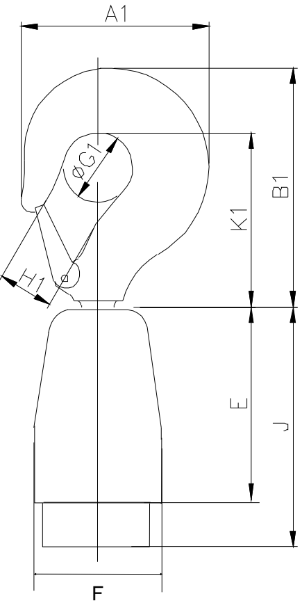
Hakenflasche
